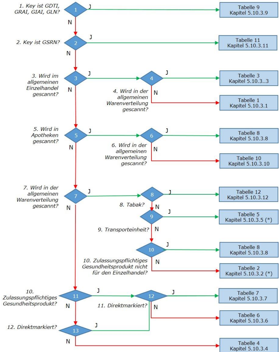
Abbildung 5.12.2.6-2. Entscheidungsbaum
